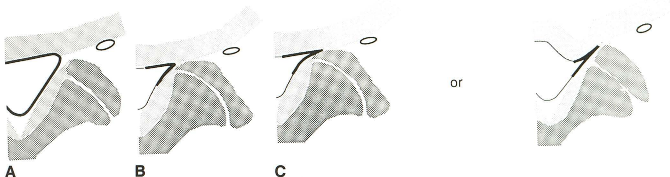
Fig. 6.—Scoring rules for AN_1 . See key for abbreviations. A, AN_1 = 1 . B, AN_1 = 3 . C, AN_1 = 5 .
